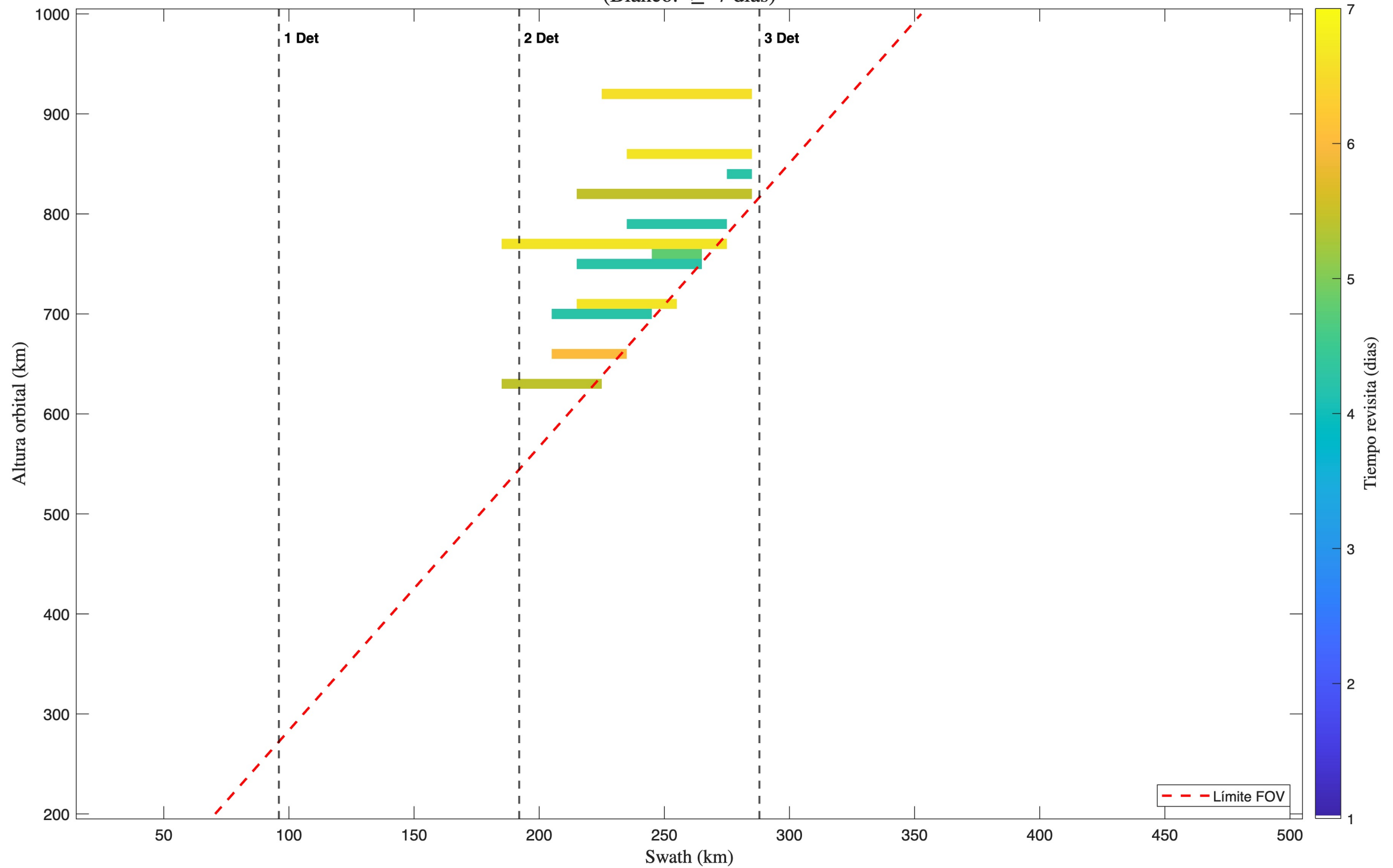
Tiempo Revisita - 2 Satellite(s); 2 Telescopio(s): Refractivo; Detector 1 (Blanco: \geq 7 días)
